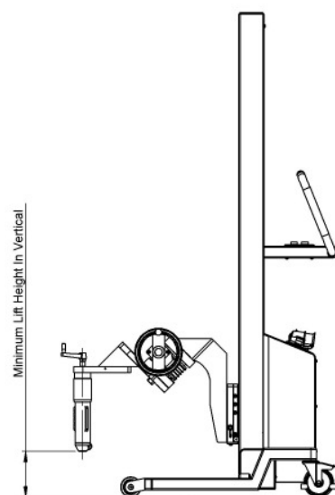
Minimális emelési magasság függőlegesen
