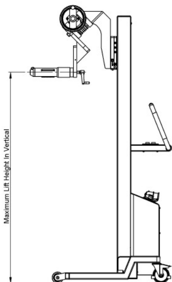
Maximális emelési magasság vízszintesen
