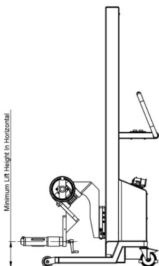
Minimális emelési magasság vízszintesen
